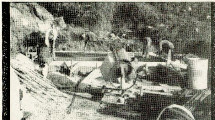
Abastecimento de água a Talhadas. Depósito de 60 m3
